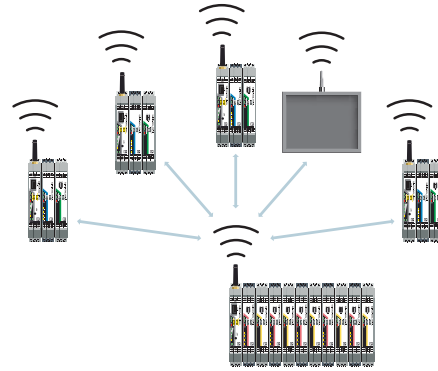
Yıldız topolojisi
